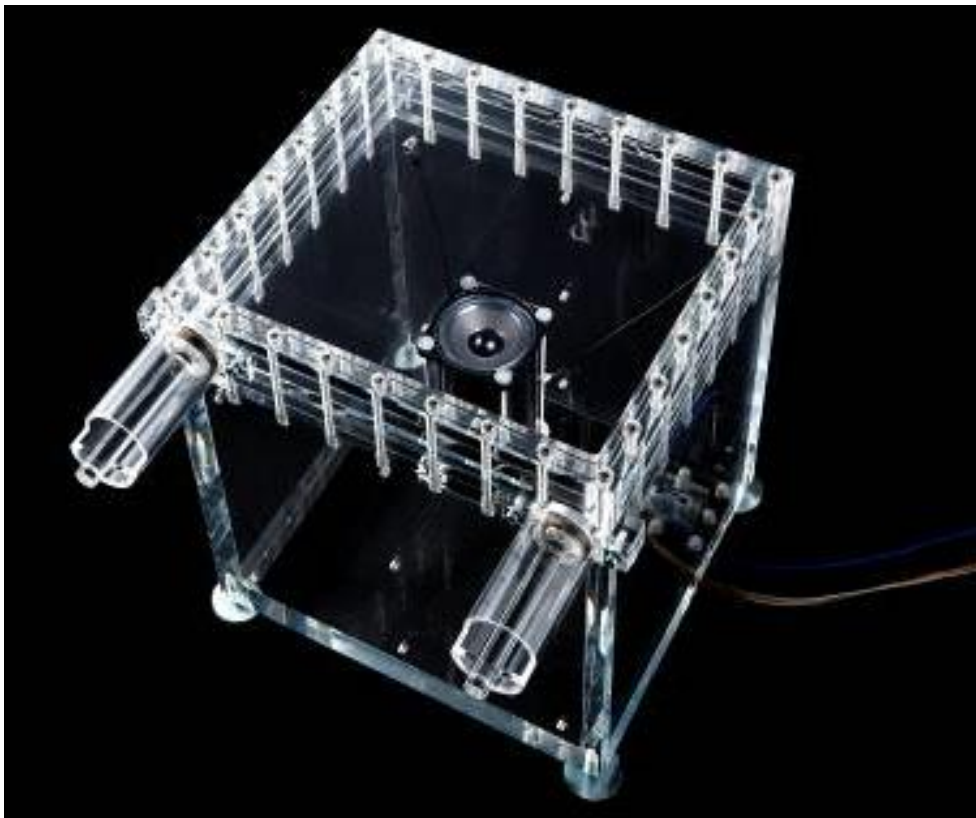
„Akustikaquarium“, bei dem zwei Helmholtz-Resonatoren die Schalltransmission eines Lautsprechers durch ein Doppelglasfenster mindern. Foto: Fraunhofer LBF
