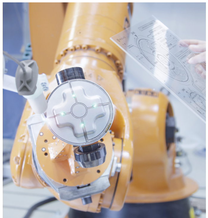
Roboter druckt eine Leiterbahn zur Ansteuerung von LEDs auf einem umgeformten Blechteil.
